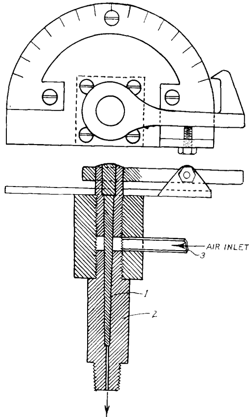
Fig. 5. Bleeder valve.
